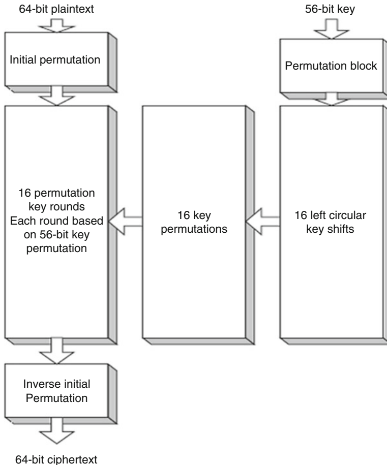
Fig. 11.3 DES algorithm
